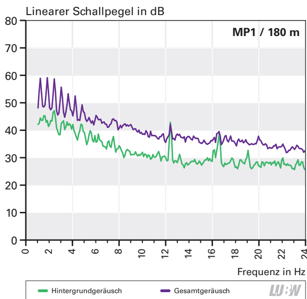
Abbildung 4.5-6: Schmalbandspektren von Hintergrundgeräusch und Gesamtgeräusch im Nahbereich der Windenergieanlage WEA 4 für den Frequenzbereich des Infrasschalls
