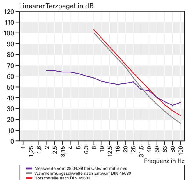
Abbildung 4.9-3: Das untersuchte Windrad erzeugt Schallwellen, die von auf einem Balkon in 250 m Entfernung stehenden Menschen nur oberhalb 40 Hz gehört werden können. Der Infrashallbereich ist hier nicht wahrnehmbar, da er deutlich unterhalb der Wahrnehmungsschwelle liegt. Quelle: [15]
