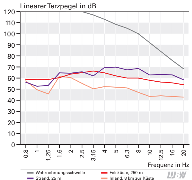
Abbildung 8.2-1: Terzspektren des Gesamtgeräusches für Meeresbrandung, unterschiedliche Randbedingungen nach [21], Wahrnehmungsschwelle nach Tabelle A3-1 zum Vergleich
