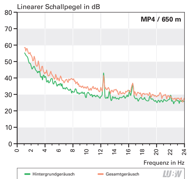
Abbildung 4.5-7: Schmalbandspektren von Hintergrundgeräusch und Gesamtgeräusch im Fernbereich der Windenergieanlage WEA 4 für den Frequenzbereich des Infrasschalls
